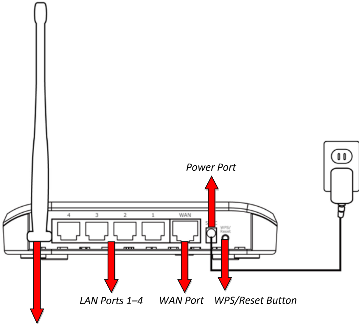
BR 6228nC V2: Detachable 3dBi Antenna X1
